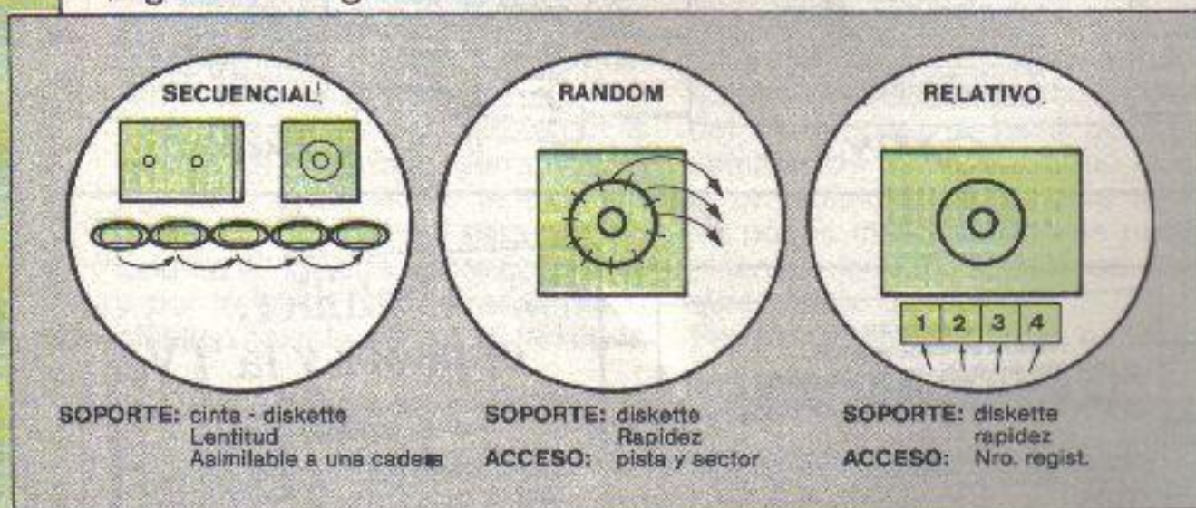
Figura 1 - Organización archivos
